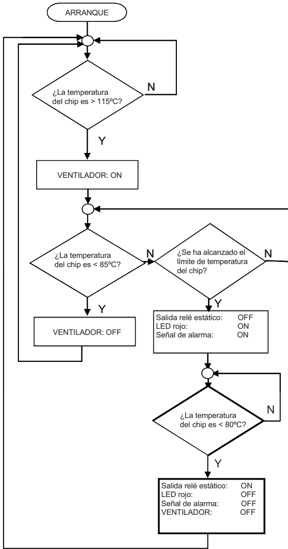
Señal de ALARMA y Ventilador (Aplicable a RGC..D92GGEP)
